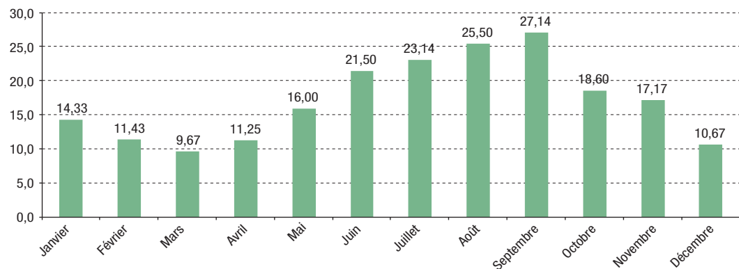
Profondeur de Secchi (exprimée en mètres)
