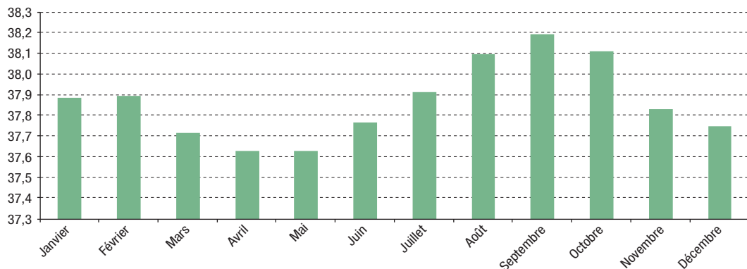
Variation mensuelle de la salinité au niveau du site de référence (exprimée en PSU)
